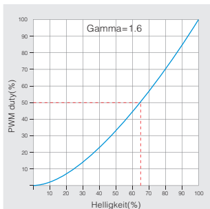
Logarithmische Dimmkurve
